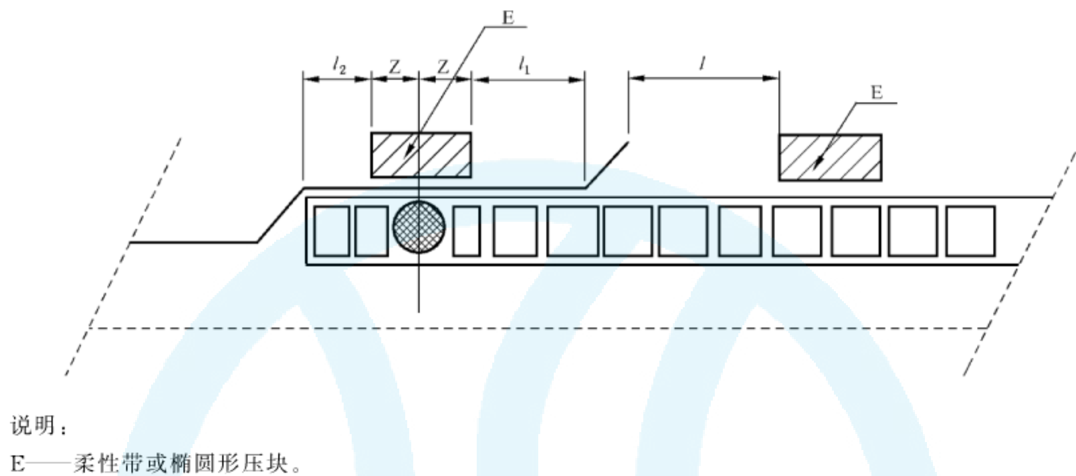
图 A.3 在连接密封处压块的定位
